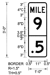
EB-MM-20 STA. 141+00
