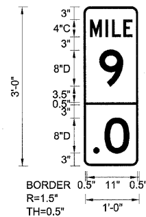
EB-MM-19 STA. 114+60
