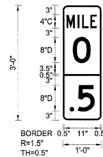
WB-MM-02 STA. 312+10
