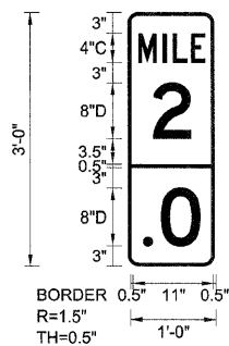
WB-MM-05 STA. 232+90
