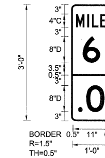
WB-MM-13 STA. 21+70
