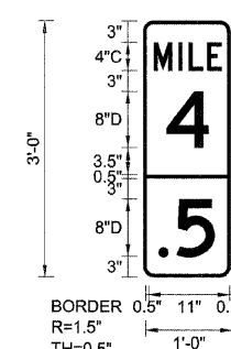
WB-MM-10 STA. 100+90
