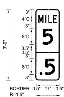
WB-MM-12 STA. 48+10
