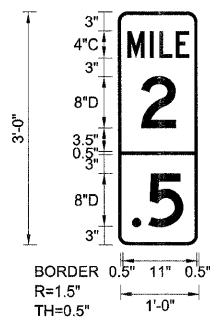
WB-MM-06 STA. 206+50
