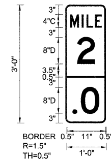
NB-MM-05 STA. 130+30
