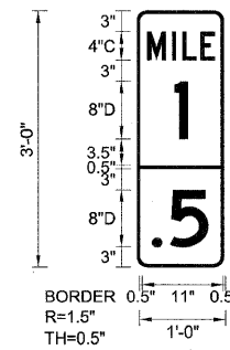
NB-MM-04 STA. 103+90
