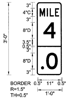
WB-MM-09 STA. 127+30
