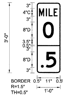
NB-MM-02 STA. 51+10
