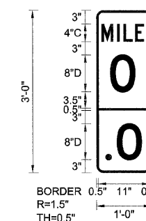
WB-MM-01 STA. 338+50
