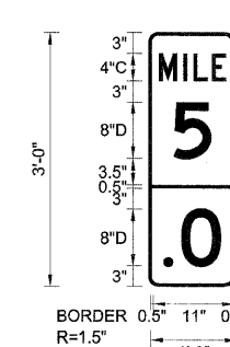
WB-MM-11 STA. 74+50
