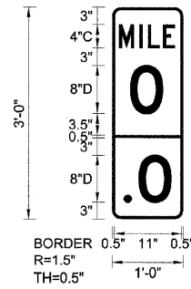
NB-MM-01 STA. 24+70
