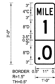
WB-MM-03 STA. 285+70
