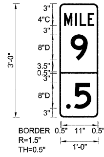
WB-MM-20 STA. 141+00
