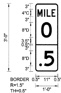
EB-MM-02 STA. 312+10
