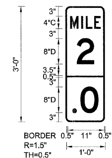
EB-MM-05 STA. 232+90
