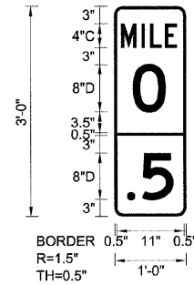
SB-MM-02 STA. 51+10
