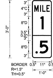
SB-MM-04 STA. 103+90
