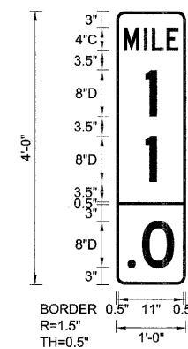
EB-MM-23 STA. 220+20
