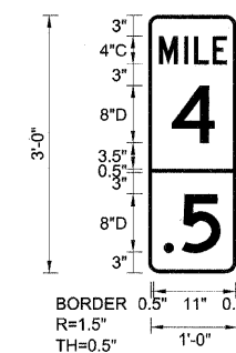
EB-MM-10 STA. 100+90
