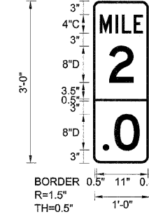
SB-MM-05 STA. 130+30
