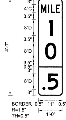
WB-MM-22 STA. 193+80
