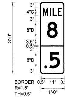
WB-MM-18 STA. 88+20
