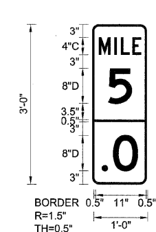
EB-MM-11 STA. 74+50
