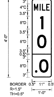
WB-MM-21 STA. 167+40
