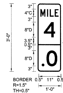
EB-MM-09 STA. 127+30
