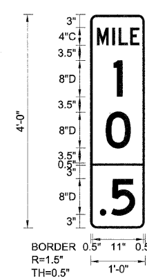
EB-MM-22 STA. 193+80
