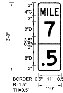
EB-MM-16 STA. 35+40
