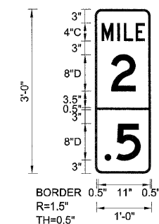
EB-MM-06 STA. 206+50
