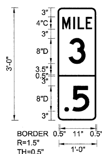
EB-MM-08 STA. 153+70
