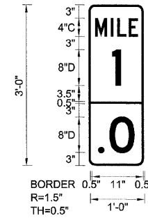
SB-MM-03 STA. 77+50
