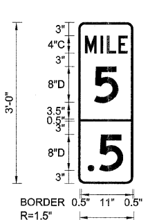
WB-MM-12 STA. 48+10
