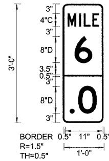
EB-MM-13 STA. 21+70
