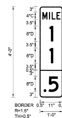
EB-MM-24 STA. 246+60
