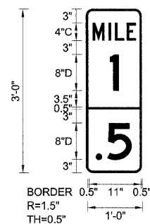
EB-MM-04 STA. 259+30
