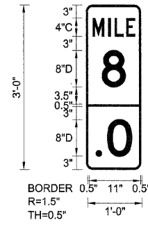
WB-MM-17 STA. 61+80
