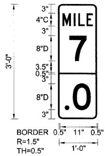
EB-MM-15 STA. 9+00
