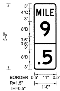
EB-MM-20 STA. 141+00
