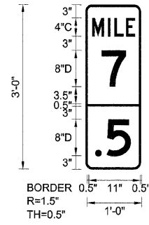
WB-MM-16 STA. 35+40
