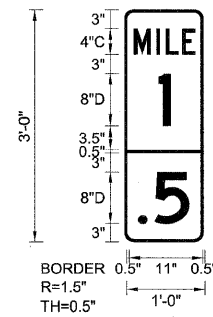
NB-MM-04 STA. 103+90
