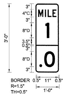
EB-MM-03 STA. 285+70
