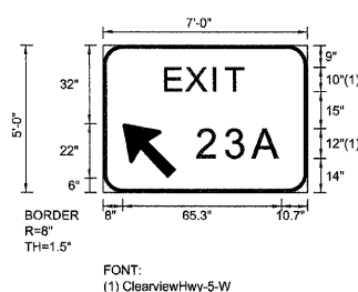
EB-WP-90 STA. 855+22
