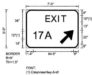
EB-WP-54 STA. 555+50
