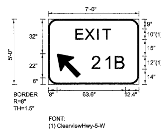
EB-WP-84 STA. 772+50
