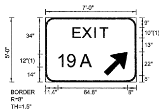
EB-WP-70 STA. 639+20
