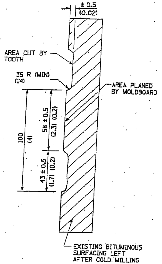
SECTION A-A
