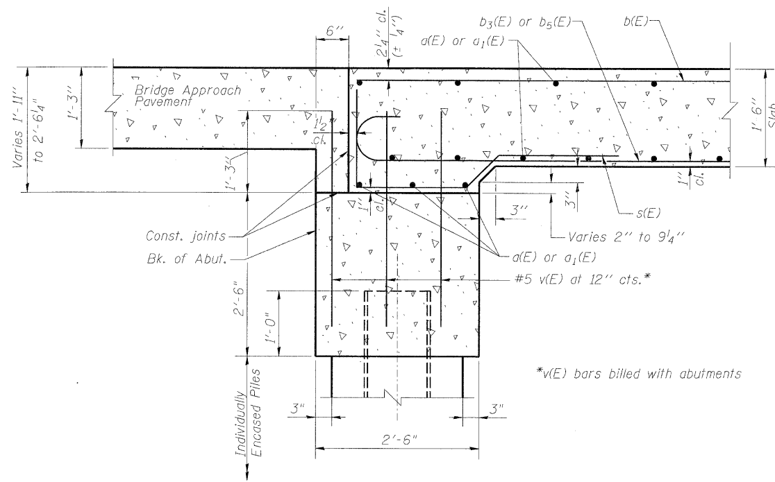
SECTION A-A
