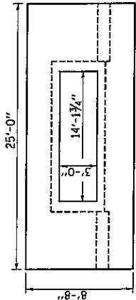
END ELEVATION
