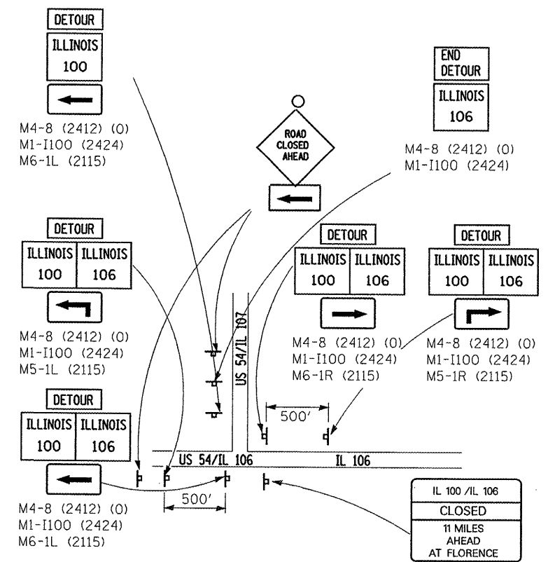
DETAIL C IL 107/IL 106 IN PITTSFIELD
