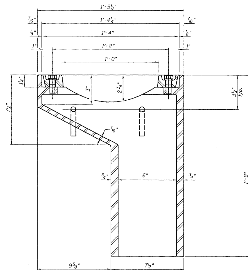
SECTION A-A
