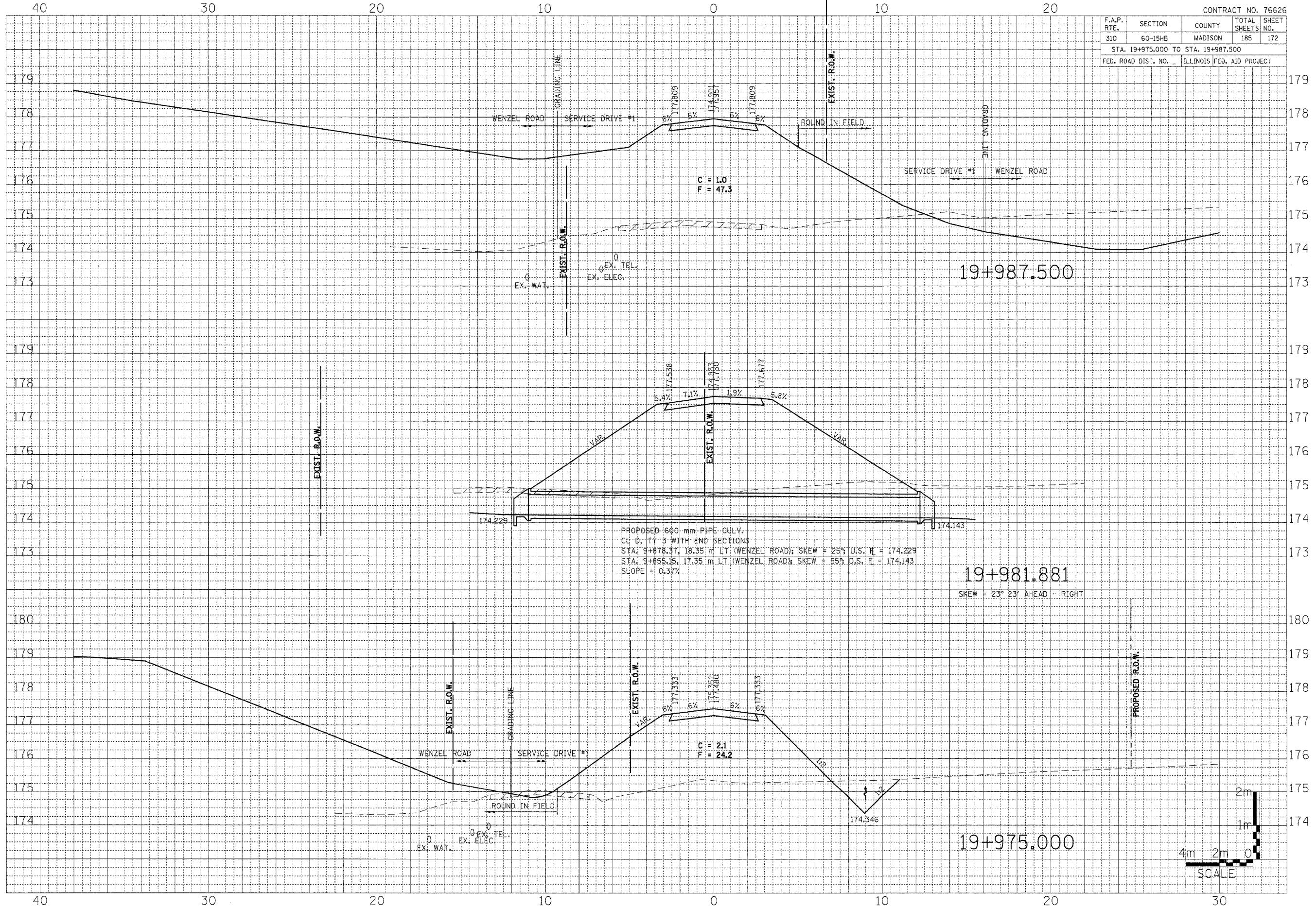
SERVICE DRIVE #1 STA. 19+975.000 TO STA. 19+987.500
