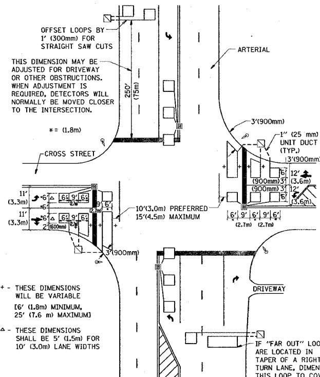
DETAIL 2 N.T.S.
