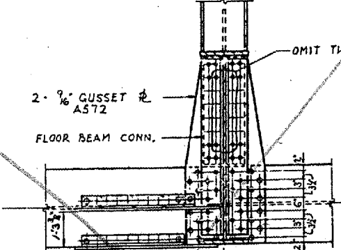
SECTION E15-E15
