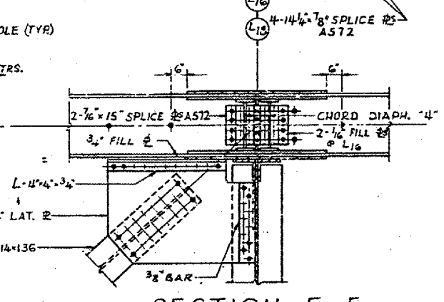
SECTION F16-F16
