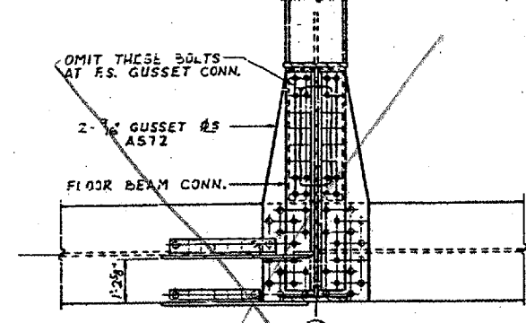
SECTION E19-E19
