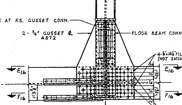
SECTION E16-E16
