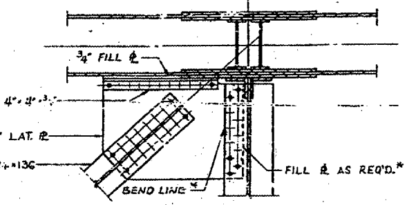
SECTION E22-E22
