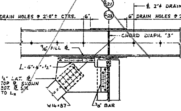
SECTION F19-F19
