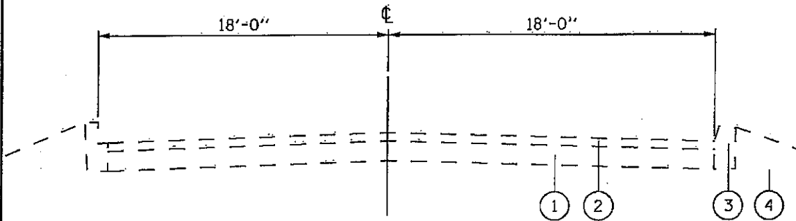
EXISTING TYPICAL SECTION STA. 140±73 TO STA. 150±91 STA. 170±01 TO STA. 188±45
