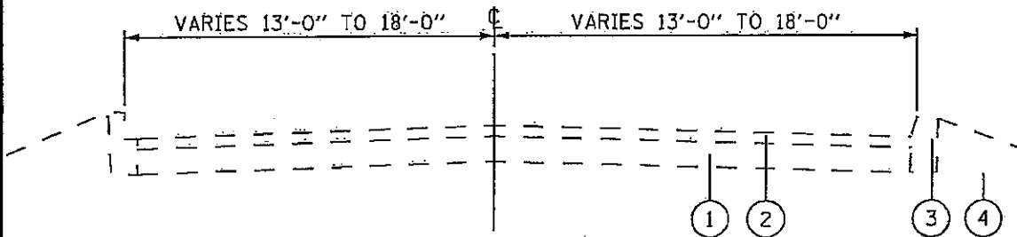
EXISTING TYPICAL SECTION STA. 150±91 TO STA. 152±72 STA. 188±45 TO STA. 188±95
