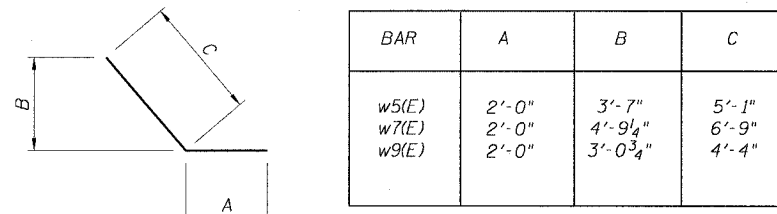
BARS w5(E), w7(E), w9(E)
