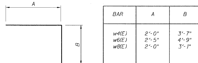
BARS w4(E), w6(E), w8(E)
