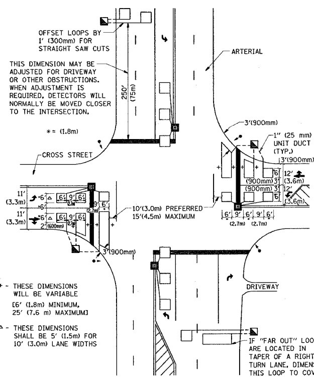
DETAIL 2 N.T.S.
