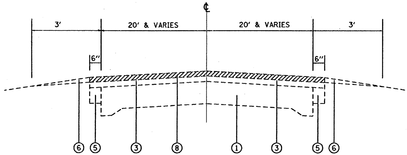
EXISTING TYPICAL SECTION STA. 29+00± TO STA. 18+90±
