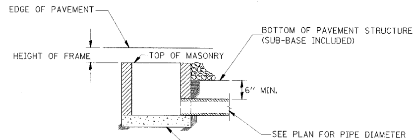
SEC. A-A
