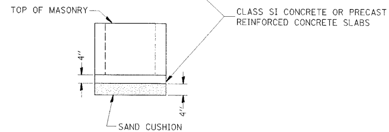
SEC. A-A
