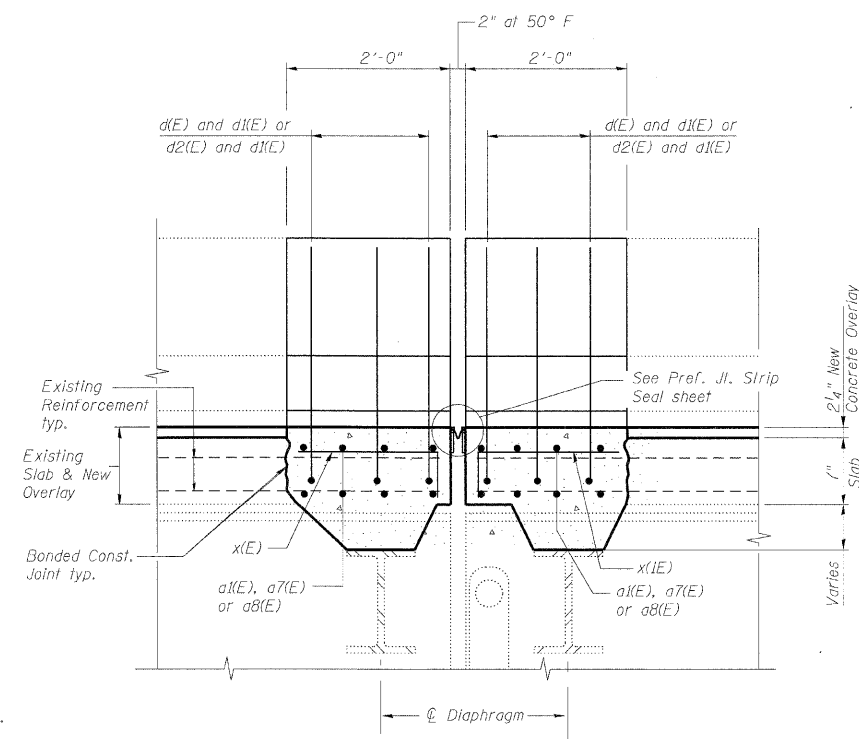
SECTION D-D
