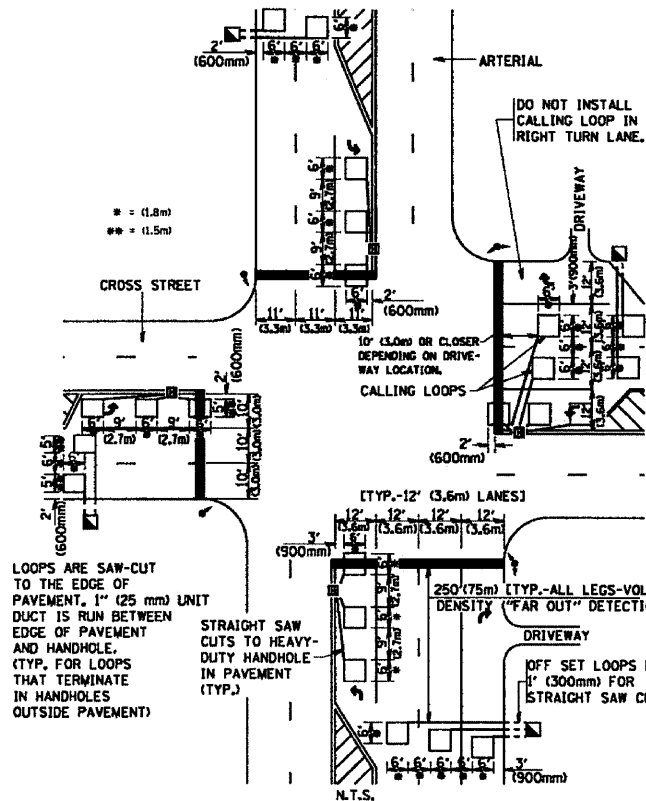
DETAIL 1 N.T.S.
