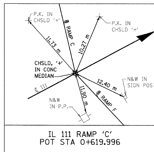
IL 111 RAMP 'C' POT STA 0+619.996 N 255,628.6235 E 697,960.6452
