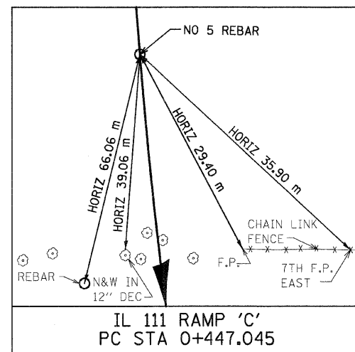
IL 111 RAMP 'C' PC STA 0+447.045 N 255,798.0981 E 697,927.1172
