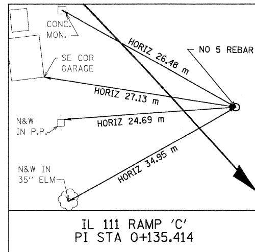
IL 111 RAMP 'C' PI STA 0+135.414 N 256,079.4320 E 697,811.2552
