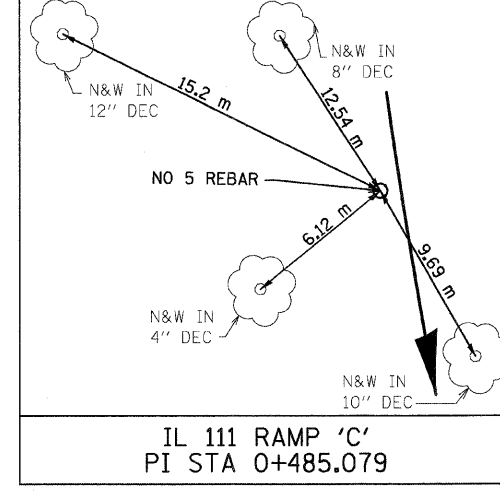
IL 111 RAMP 'C' PI STA 0+485.079 N 255,760.1795 E 697,930.0789
