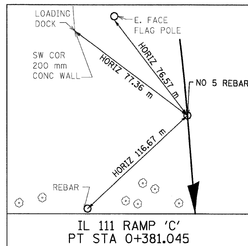
IL 111 RAMP 'C' PT STA 0+381.045 N 255,863.8976 E 697,921.9778
