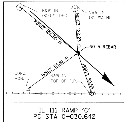
IL 111 RAMP 'C' PC STA 0+030.642 N 256,148.7703 E 697,732.7103
