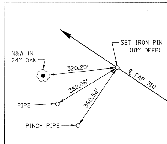
FAP 310 (IL 255) PT STA 105+37.40
