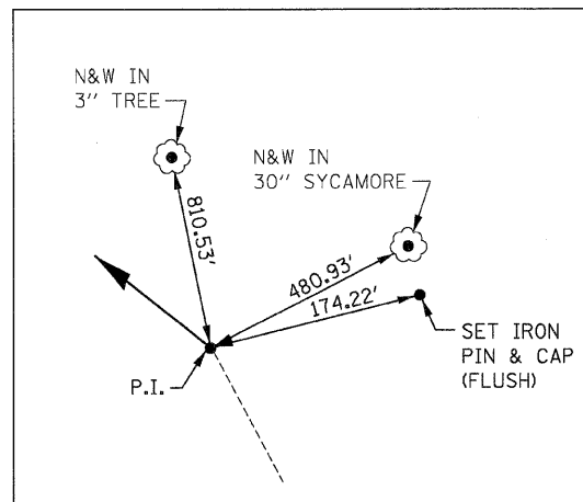
FAP 310 (IL 255) PI STA 80+34.80
