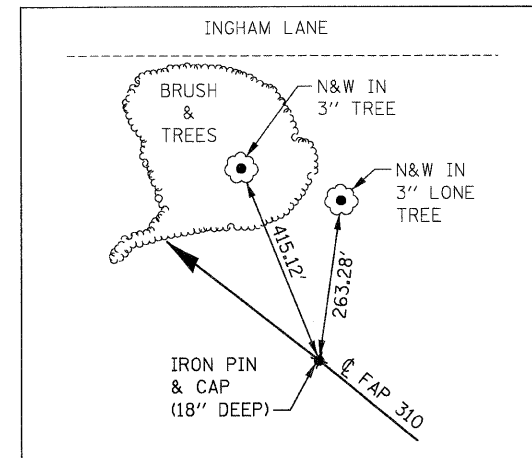
FAP 310 (IL 255) PT STA 87+00.91
