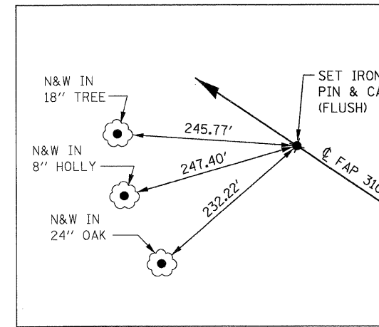
FAP 310 (IL 255) PC STA 107+41.67
