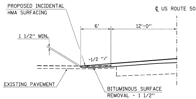
SECTION DETAIL G-G CL STA. 108+40
