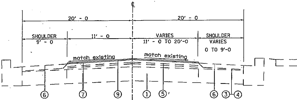
IL RTE 100 TYPICAL MI STA. 19.84 TO MI STA. 19.90
