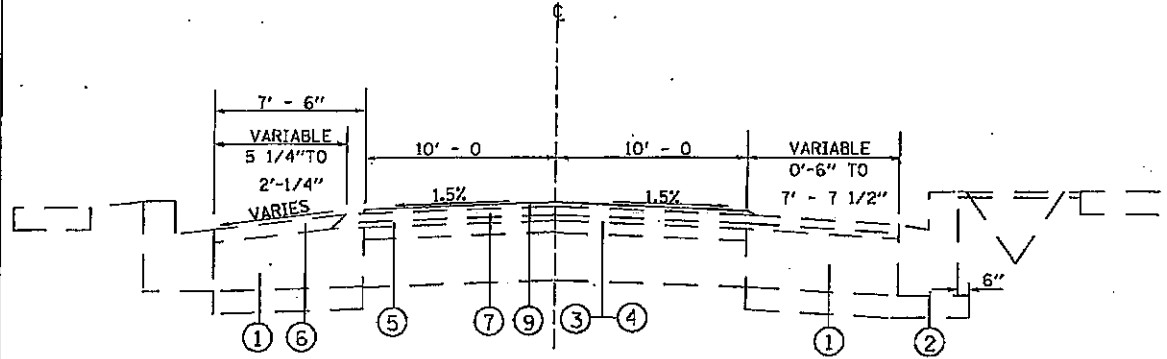
IL RTE 100 TYPICAL MI STA. 19.77 TO MI STA. 19.82
