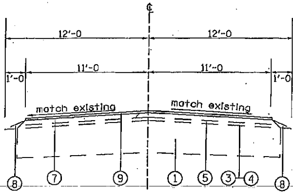
IL RTE 100 TYPICAL MI STA. 18.51 TO MI STA. 19.77
