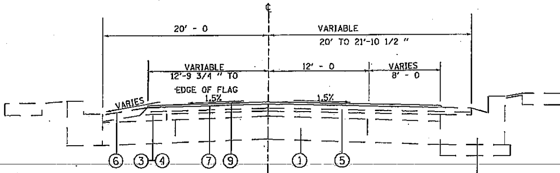
IL RTE 100 TYPICAL MI STA. 19.83 TO MI STA. 19.84
