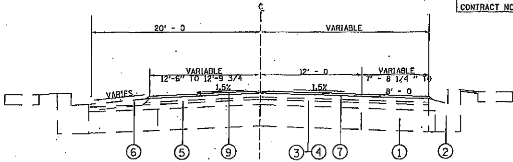
IL RTE 100 TYPICAL MI STA 19.82 TO MI STA. 19.83
