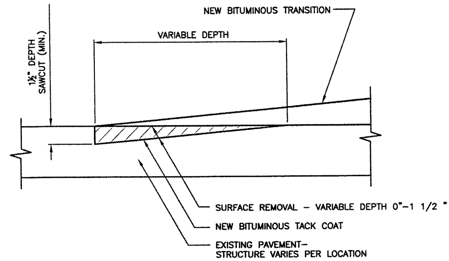
BUTT JOINT DETAIL N.T.S.
