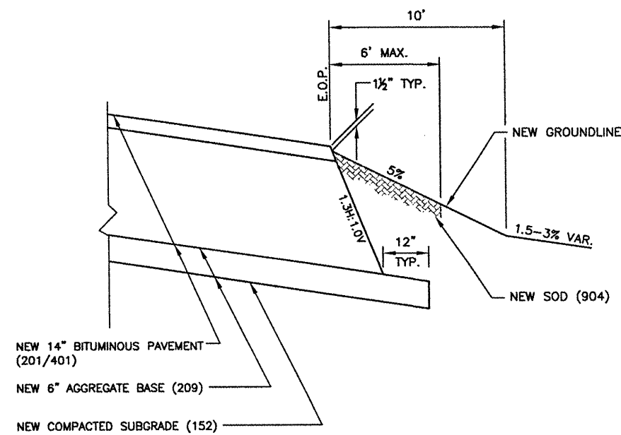
NEW SHOULDER DETAIL "B" N.T.S.
