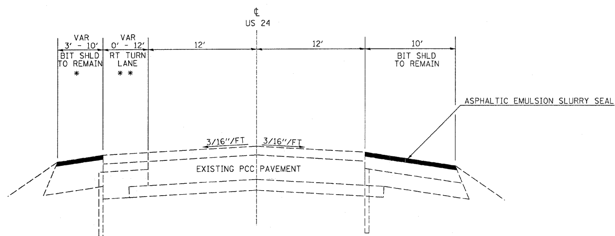
TYPICAL SECTION #3 STA 3016+25 TO STA 3021+75 STA 3030+50 TO STA 3036+50
