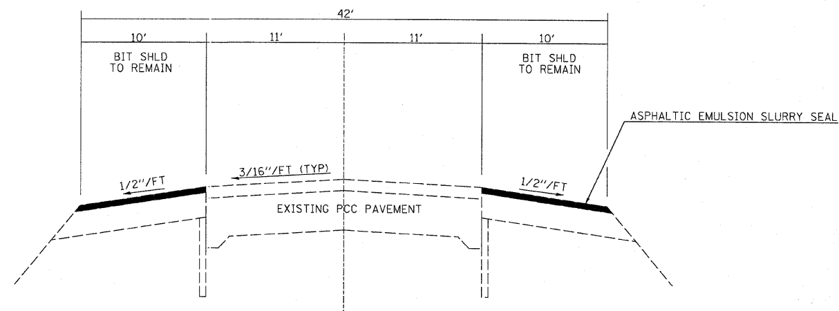
TYPICAL SECTION #4 STA 3037+42 - STA 3042+83
