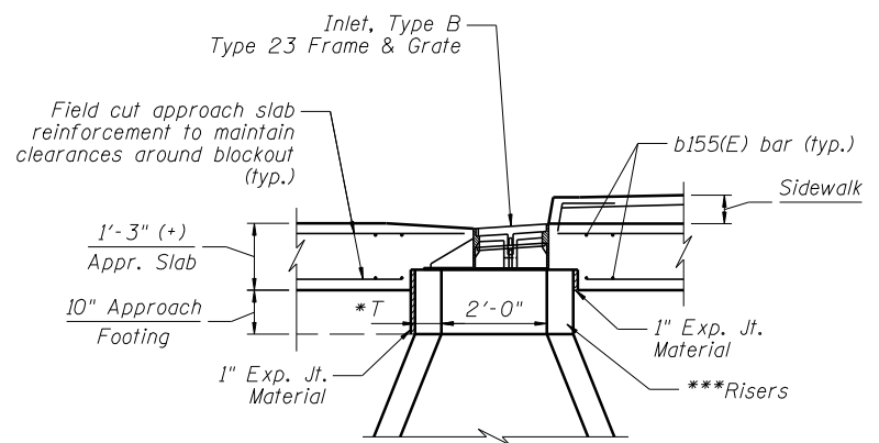
SECTION AA-AA
