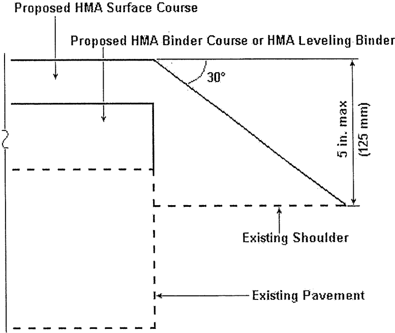
Safety Edge at Edge of Pavement
