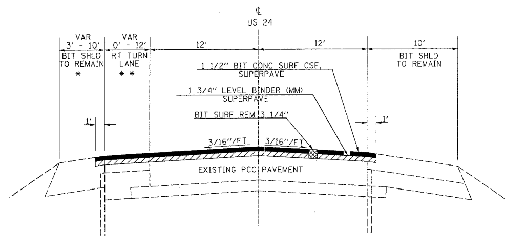
TYPICAL SECTION STA 3016+25 TO STA 3021+75 STA 3030+50 TO STA 3036+50
