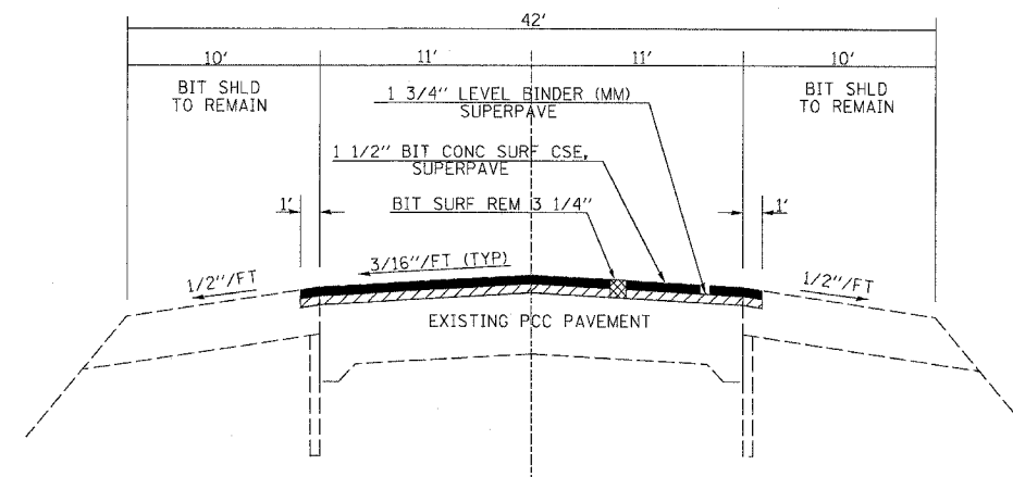
TYPICAL SECTION STA 3037+42 - STA 3042+83
