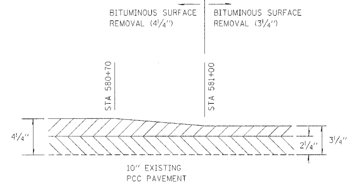
MILLING TRANSITION DETAIL STA. 580+70 TO STA. 581+00 *
