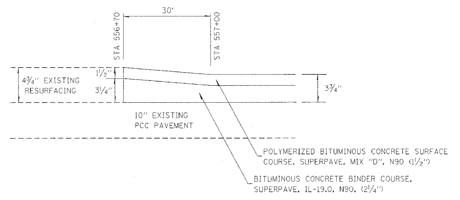
BUTT JOINT DETAIL STA. 556+70 TO STA. 557+00
