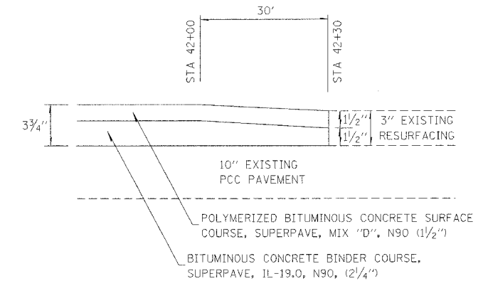
BUTT JOINT DETAIL STA. 42+00 TO STA. 42+30
