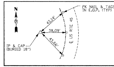
STA EQUATION PT STA 1115+51.02 BK = STA 1116+02.92 AH
