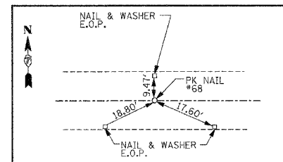
TR1550N STA 5+00.00 PK NAIL #68
