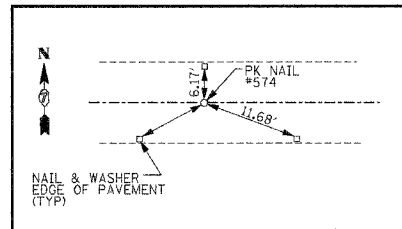
TR1725N STA 5+00.00 PK NAIL #574
