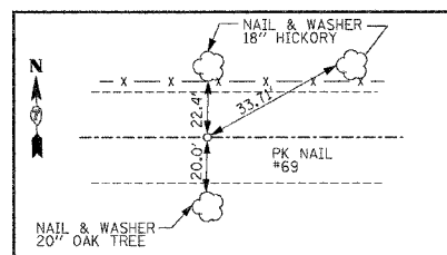
TR1550N STA 15+00.00 PK NAIL #69
