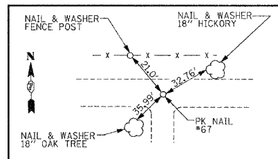
TR1625N STA 15+00.00 PK NAIL #67
