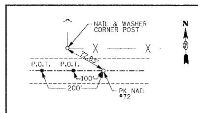
TR1500N STA 15+00.00 PK NAIL #72
