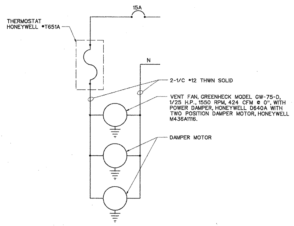
VENT FAN AND DAMPER WIRING
