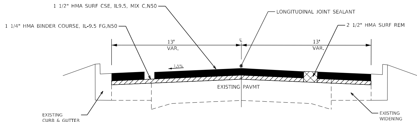
TYPICAL SECTION 6 STA 36+49 TO STA 25+77
