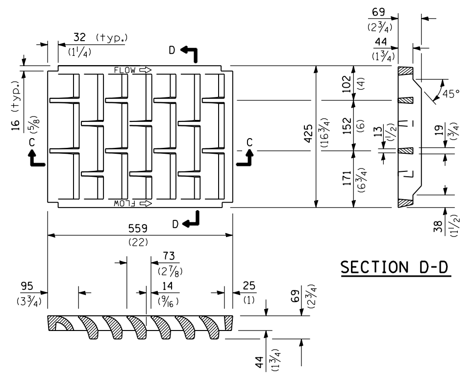
SECTION D-D
