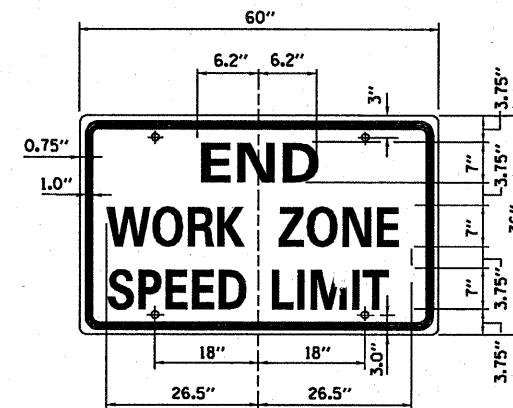
SIGN G20-1103
