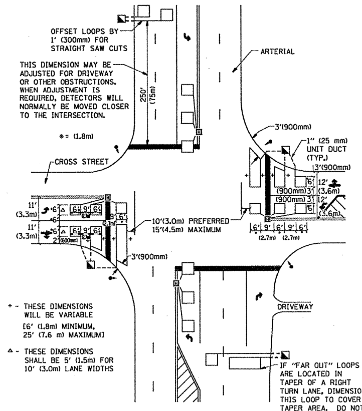
DETAIL 2 N.T.S.
