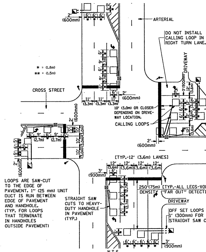
DETAIL 1 N.T.S.
