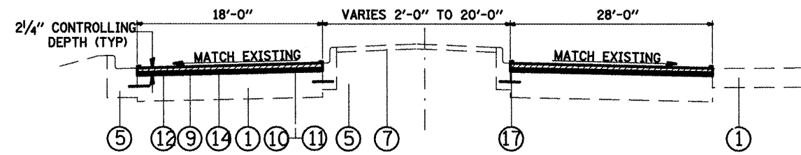
TYPICAL SECTION STA. 13+33 TO STA. 14+11
