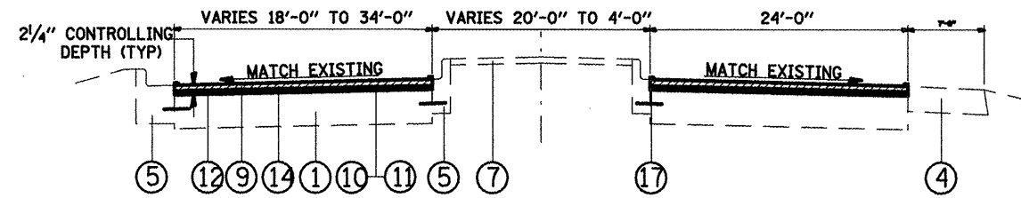
TYPICAL SECTION STA. 10+30 TO STA. 11+71
