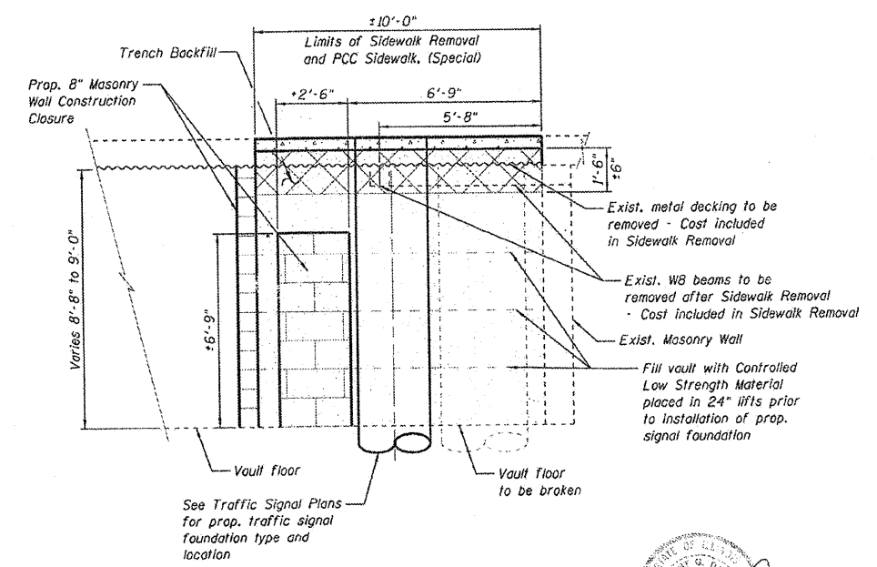
SECTION D-D
