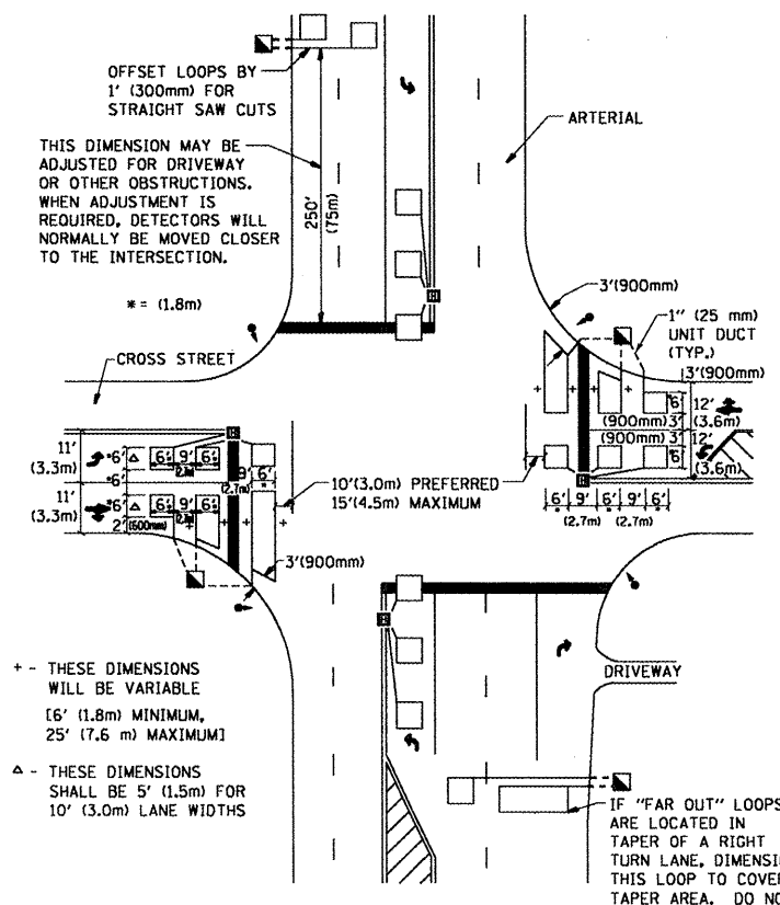
DETAIL 2 N.T.S.
