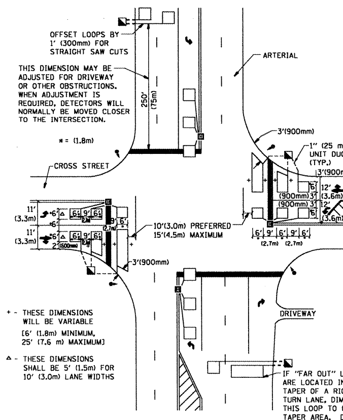
DETAIL 2 N.T.S.
