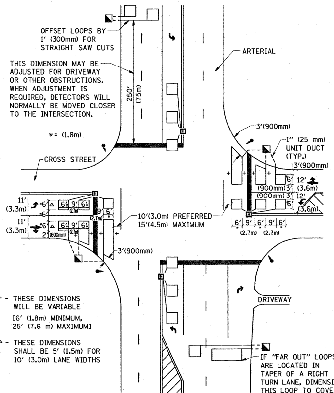
DETAIL 2 N.T.S.
