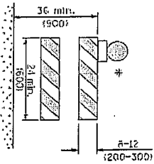
TYPE II BARRICADE
