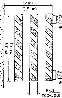
TYPE III BARRICADE
