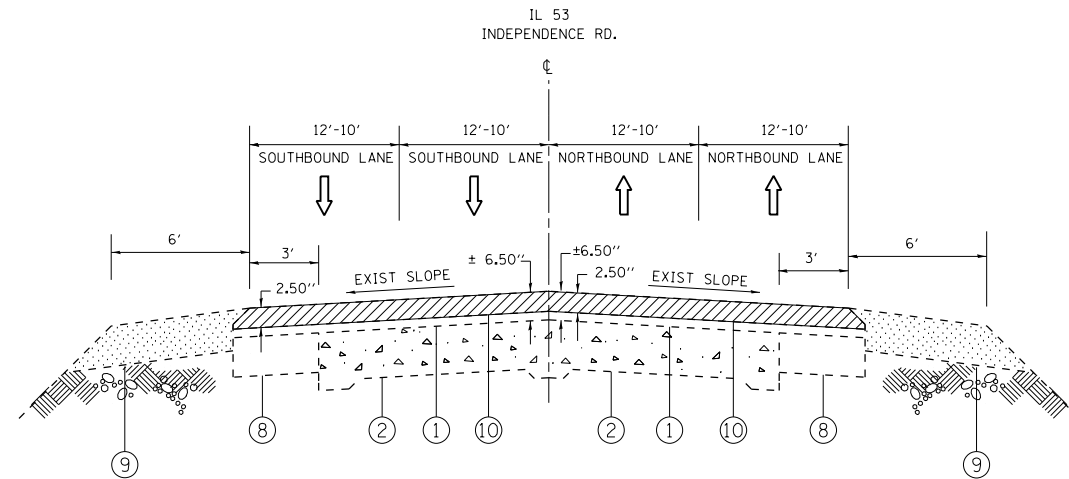
IL 53 (INDEPENDENCE RD) EXISTING TYPICAL SECTION STA. 14+49 TO STA. 60+00 STA. 73+67 TO STA. 114+53 STA. 127+20 TO STA. 149+04
