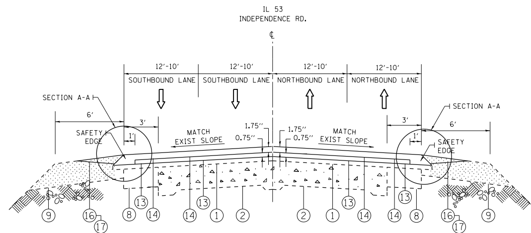
IL 53 (INDEPENDENCE RD) PROPOSED TYPICAL SECTION STA. 14+49 TO STA. 60+00 STA. 73+67 TO STA. 114+53 STA. 127+20 TO STA. 149+04
