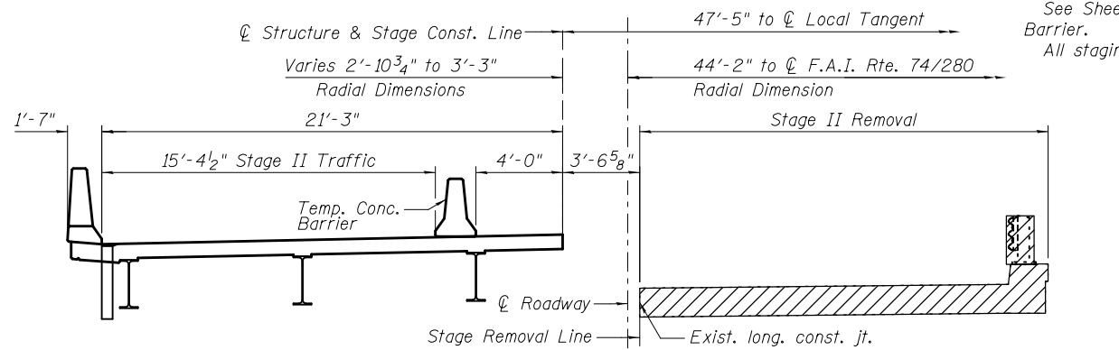
STAGE II REMOVAL: SN 081-0195 (W.B.)
