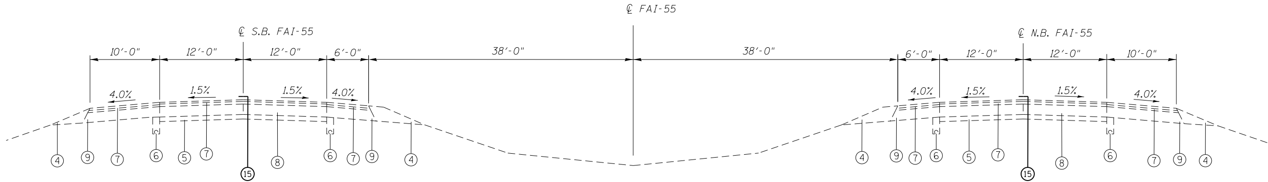
TYPICAL #21 S.B. & N.B. FAI-55 STA. 429+92.22 TO STA. 453+88.01 STA. 477+74.85 TO STA. 513+89.55 STA. 539+22.87 TO STA. 549+92.23
