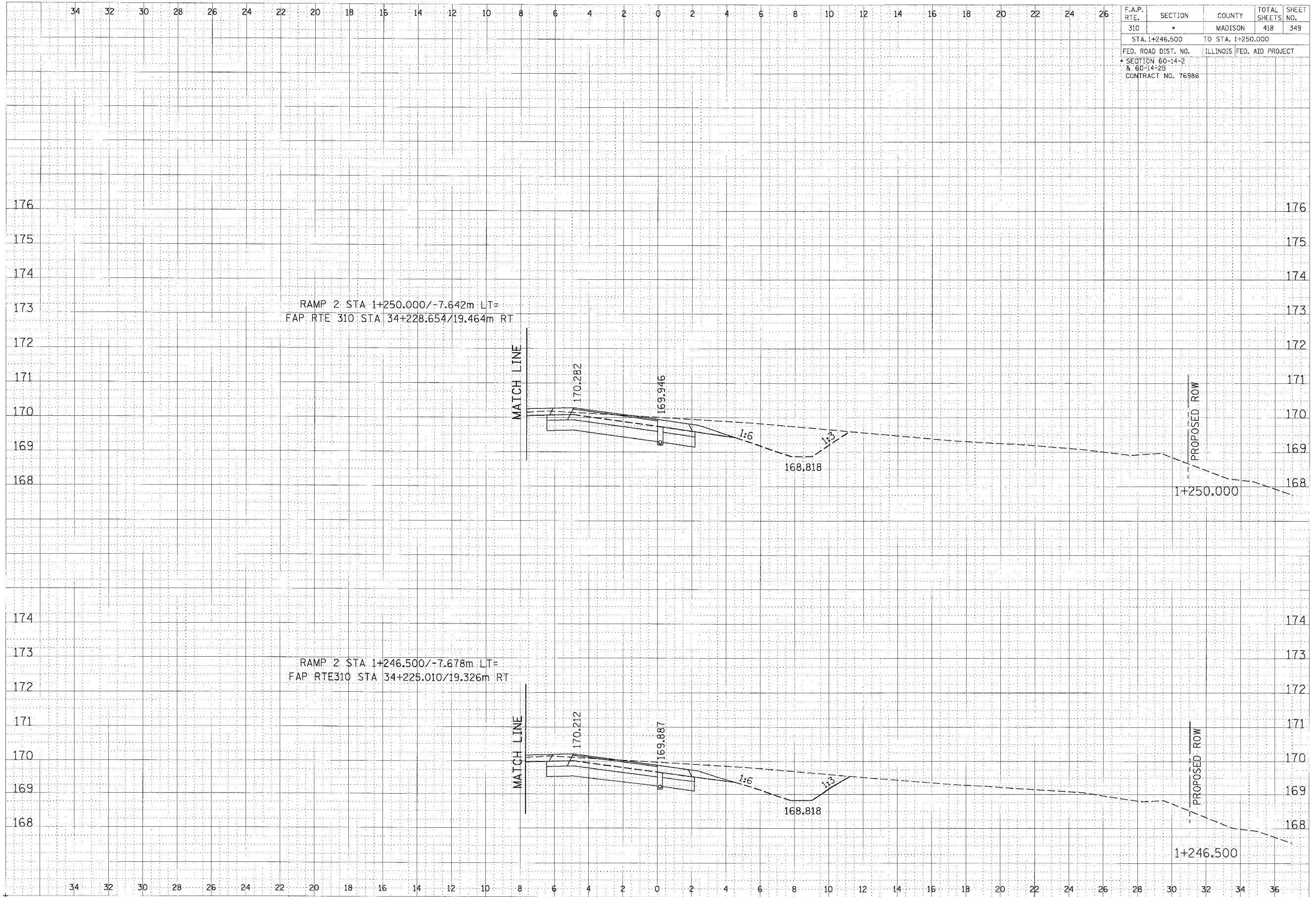
RAMP 2 CROSS SECTION, STA 1+246.500 TO STA 1+250.000
