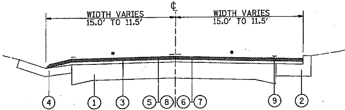
TYPICAL SECTION ① STA 1+45 TO STA 4+34
