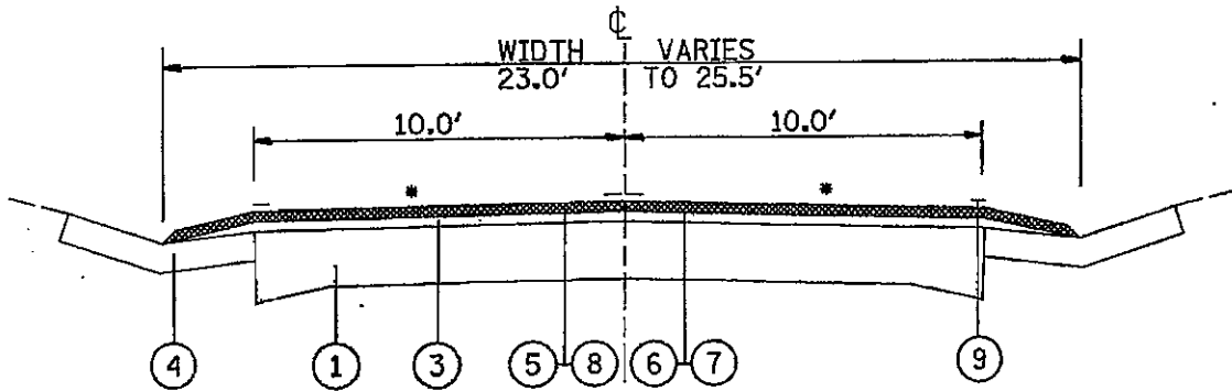
TYPICAL SECTION ② STA 4+34 TO STA 19+89 OMISSION STA 19+89 TO STA 38+55
