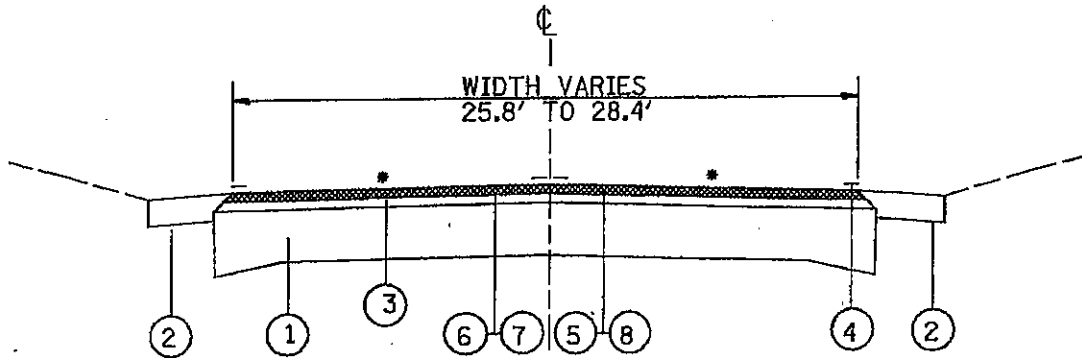
TYPICAL SECTION 3 STA 38+55 TO STA 39+55 STRUCTURE OMISSION STA 38+55 TO STA 38+89
