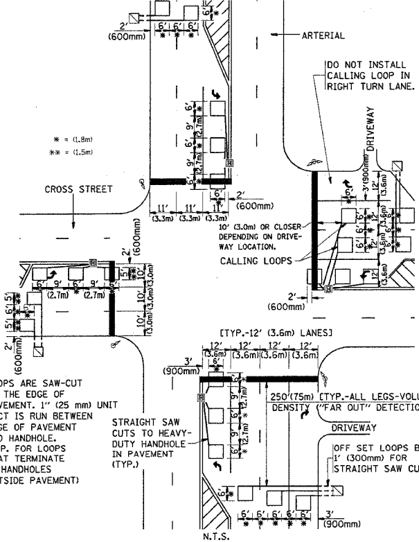
DETAIL 1 N.T.S.
