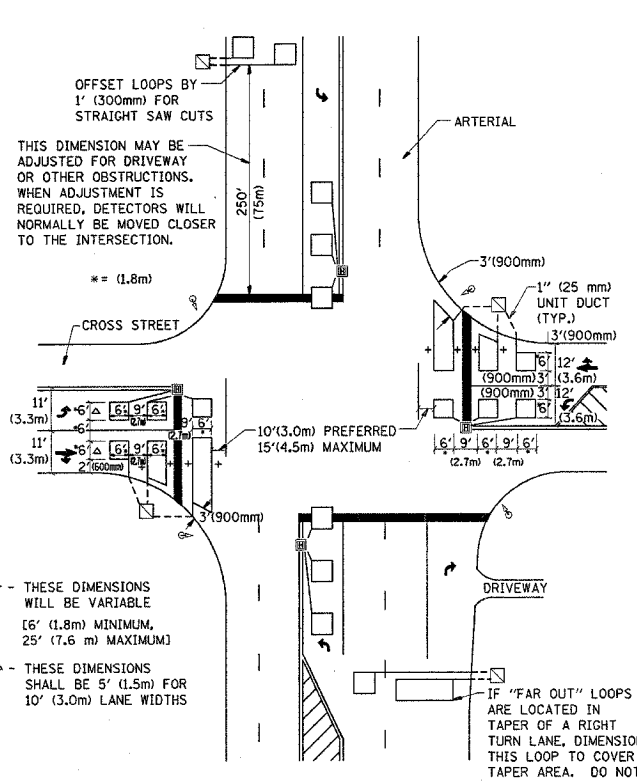
DETAIL 2 N.T.S.
