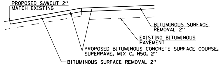
SECTION A-A @ STA 681+00 LT & RT
